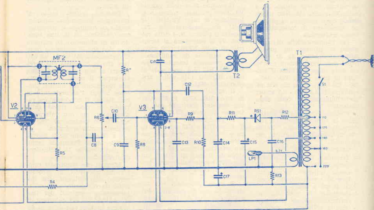
Fig. 1. — SCHEMA ELETTRICO
