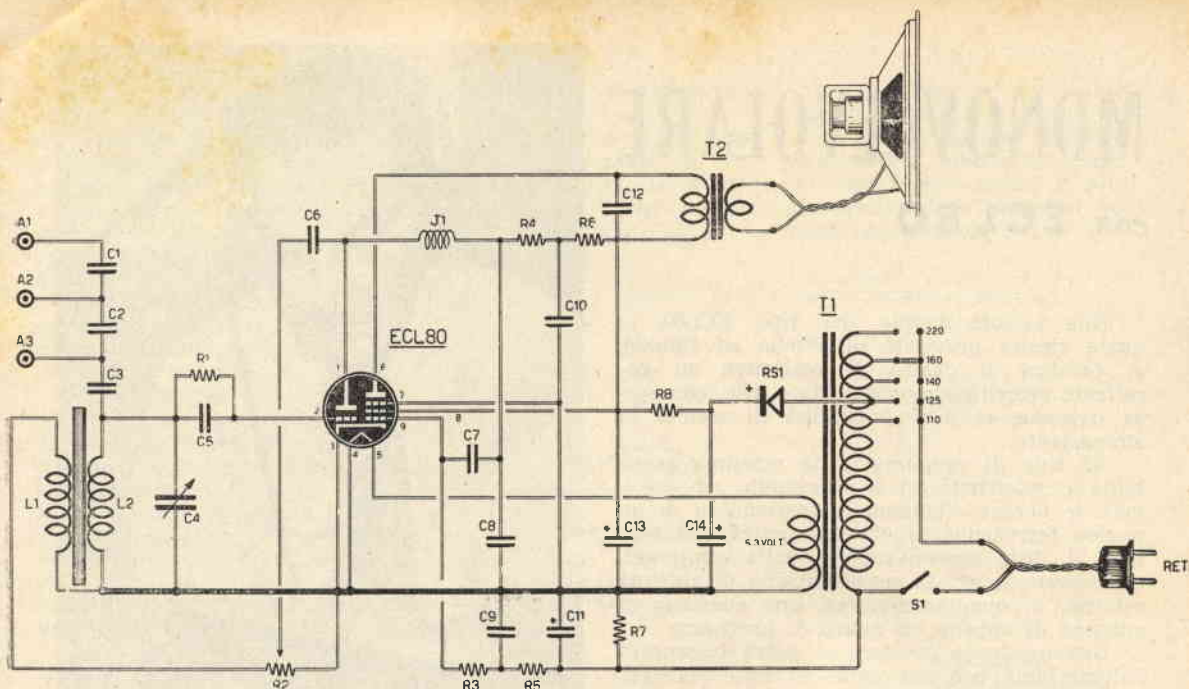
Fig. 1. — Schema elettrico.
